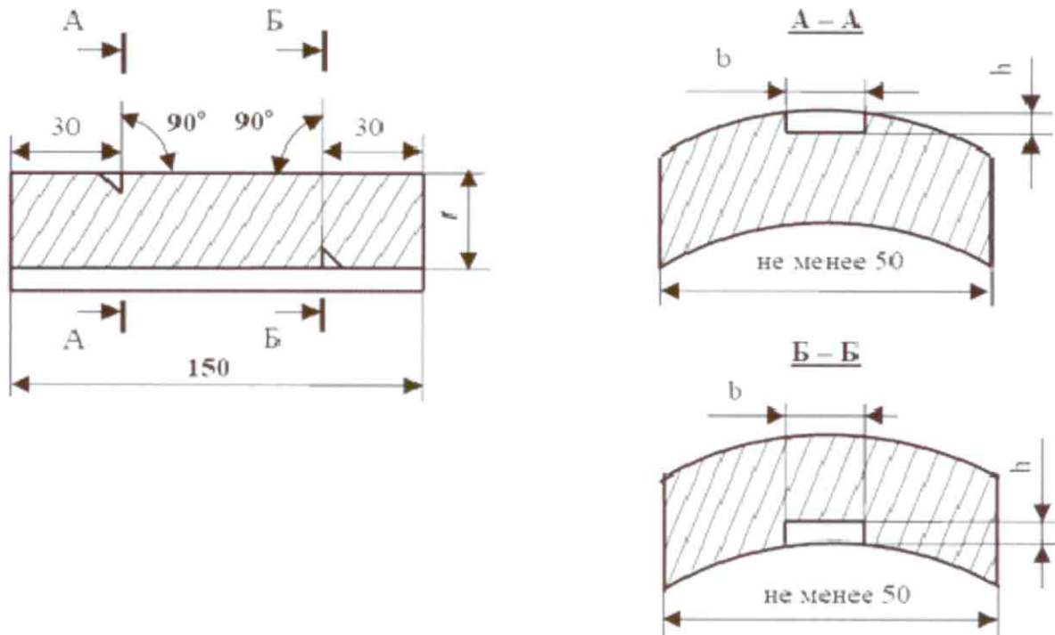
Рисунок 2 - Чертеж СОП для настройки браковочного уровня
