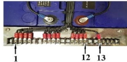
J4 - разъем подключения блока управления тележки АКБ
