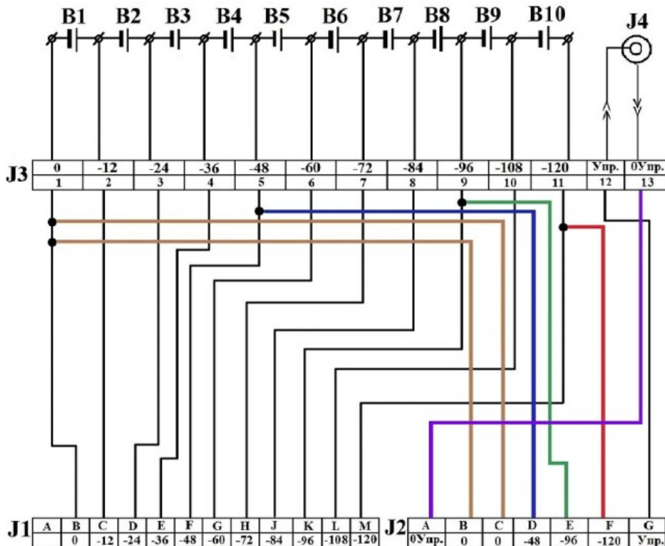
Схема электрическая аккумуляторного блока (АКБ) С-300М
