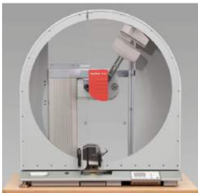
Рисунок 3 – Общий вид копров маятниковых HIT25P, HIT50P
