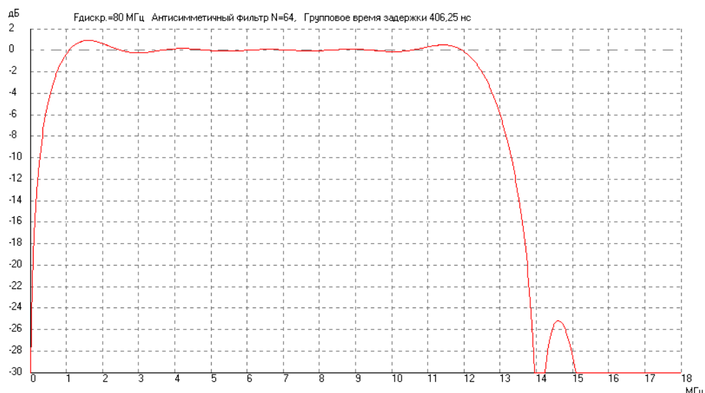
Рис. 4.4.3. Амплитудно-частотная характеристика цифрового фильтра высоких частот 0,8 – 12 МГц.
