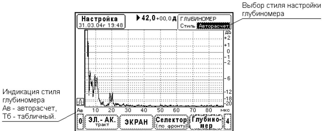
Рис. 9.4.4.1. Выбор стиля настройки глубиномера.
